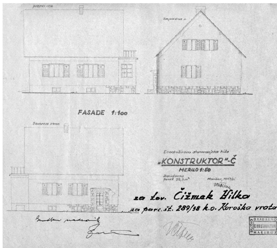
Slika 2: Fragment načrta Konstruktorjeve enodružinske stanovanjske hiše Čižmekovih na Pasterkovi 4, zazidalna površina 93,9 m 2 , Maribor, 1950/Si. Merilo načrta 1:50, merilo za fasado 1:100, format: 888 × 573 mm. Hrani PAM, fond Pasterkova 4.
